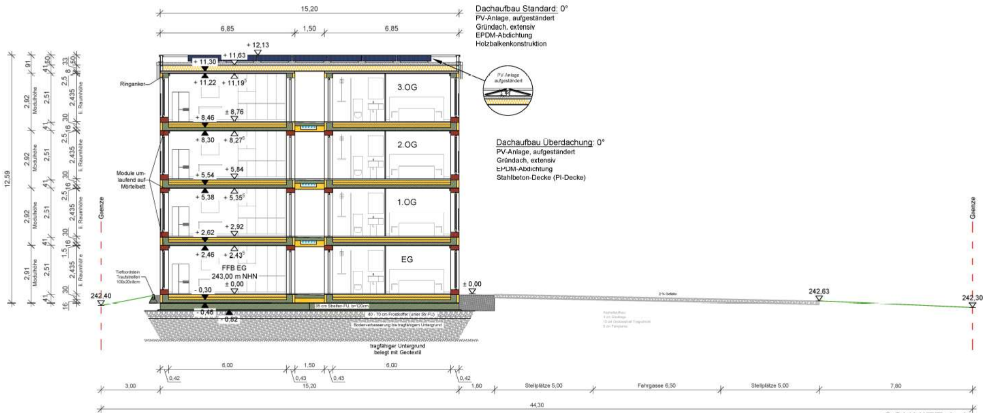
SCHNITT A-A
